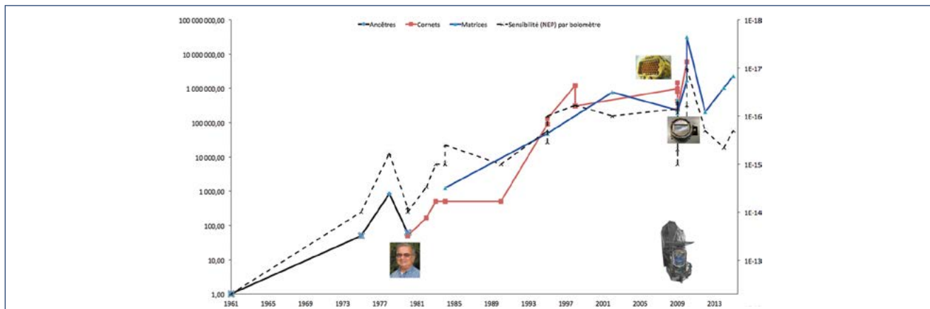
Figure 2. Diagramme schématisant des lignées techniques des bolomètres, les premiers modernes qualifiés d'ancêtres, puis la lignée à cornets, débutant quelques années après l'invention des cônes de R. Winston en 1970, et enfin celle des bolomètres organisés en matrices. Le niveau de performance (à gauche en ordonnée) est le nombre de bolomètres (dans l'instrument) multiplié par l'efficacité (ouverture efficiency) divisé par la sensibilité (Noise Equivalent Power, NEP) des bolomètres individuels. Ce niveau de performance permet de comparer des caméras de bolomètres. Les courbes de performances des lignées "cornets" et "matrices" se rejoignent en 2009 avec les instruments SPIRE et PACS du satellite Herschel. À titre comparatif, la courbe hachurée représente l'évolution du NEP (à droite en ordonnée). Les photos de R. Winston et des instruments sont placées sur la chronologie.
